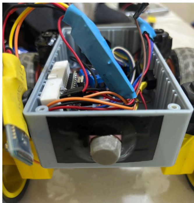
Figura 2 Vista del Sistema de Detección de Gas
